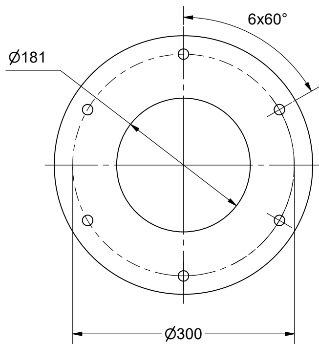
PE Sheet ( 1 : 5 )
