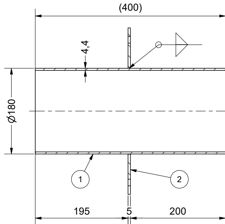
A-A ( 1 : 5 )
